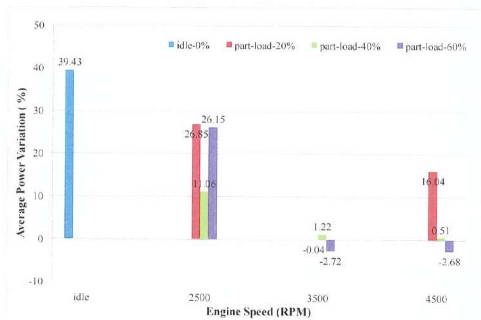
圖 1-2、在不同轉速下與不同負載下比較使用 HG668 機油添加劑產品前與之後對輸出功率(Power)之平均變化率
