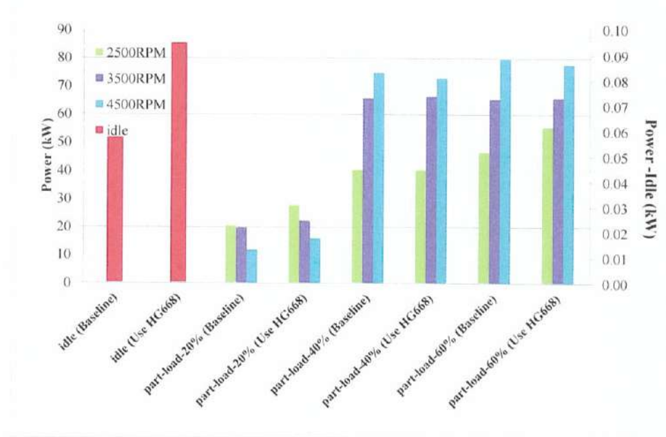
圖 1-1、在不同轉速下與不同負載下比較使用 HG668 機油添加劑產品前與之後對輸出功率(Power)影響
